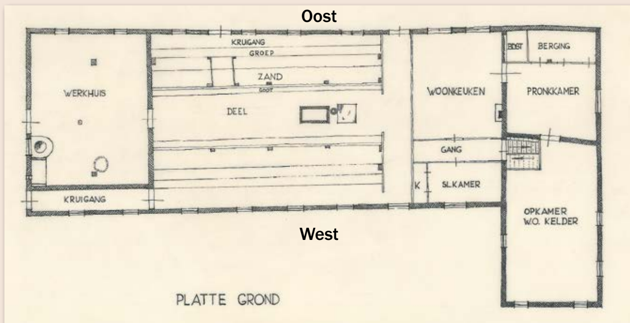
afb. 3 Plattegrond (oostgevel is boven).
